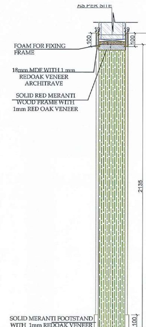
FRAME DETAIL SECTION (A-A) SCALE: 1:5
