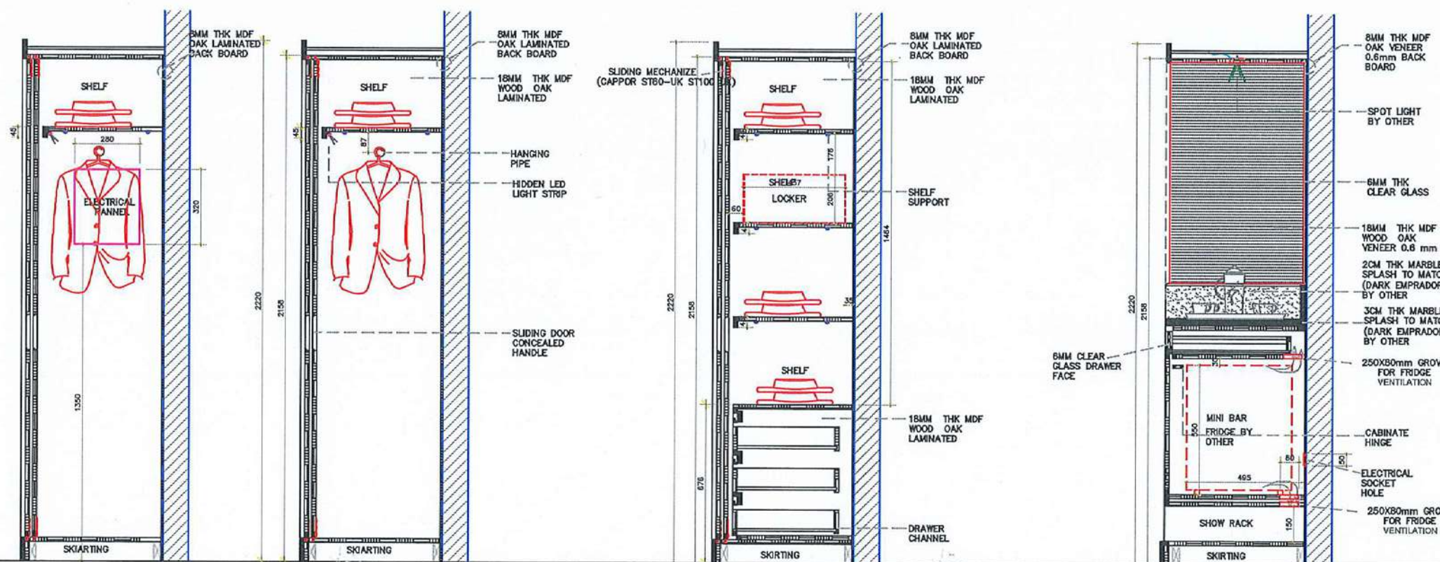
CLOSET WITH MINI BAR SECTION D-D
