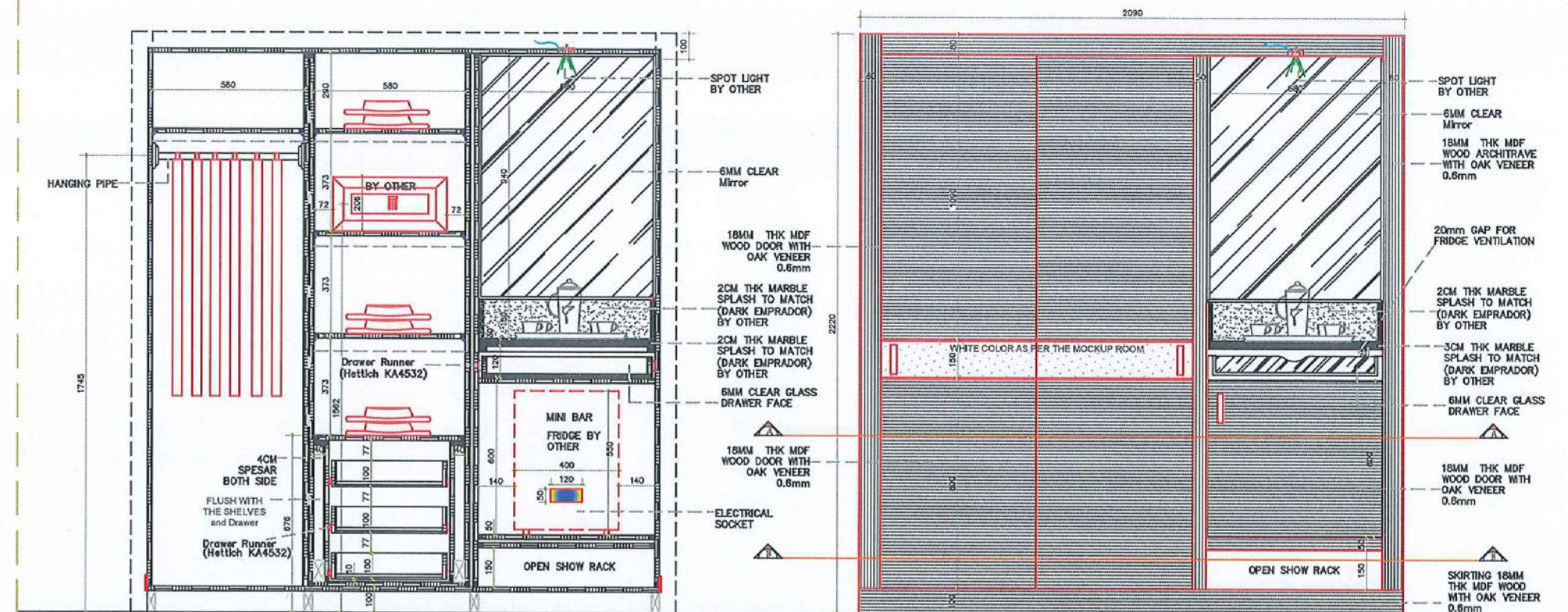
CLOSET WITH MINI BAR OPEN ELEVATION
